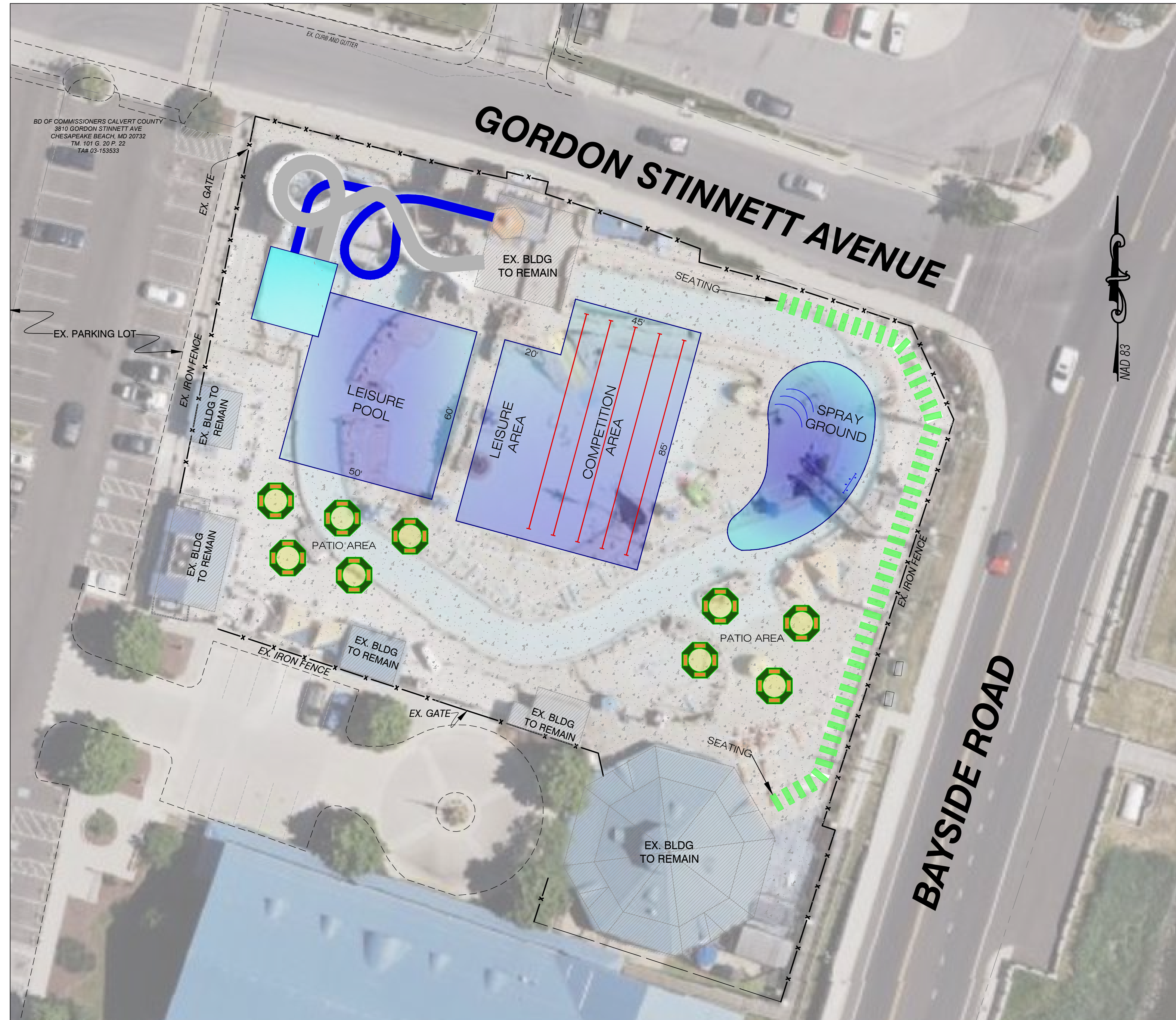
PLAN SCALE: 1" = 20'
